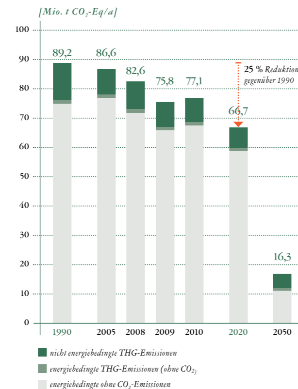
ENTWICKLUNG DER THG-EMISSIONEN BIS 2020 NACH DEM KLIMASCHUTZZIEL FÜR BADEN-WÜRTTEMBERG (BASIS: ENERGIESZENARIO 2050)
